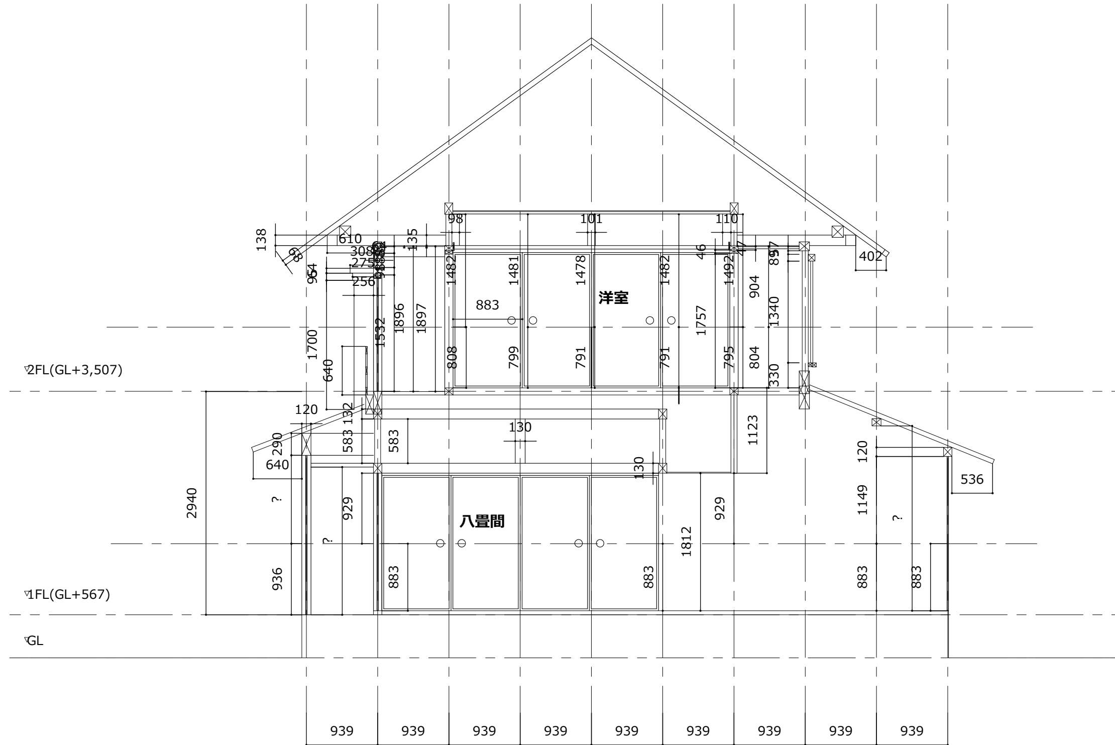
断面図
