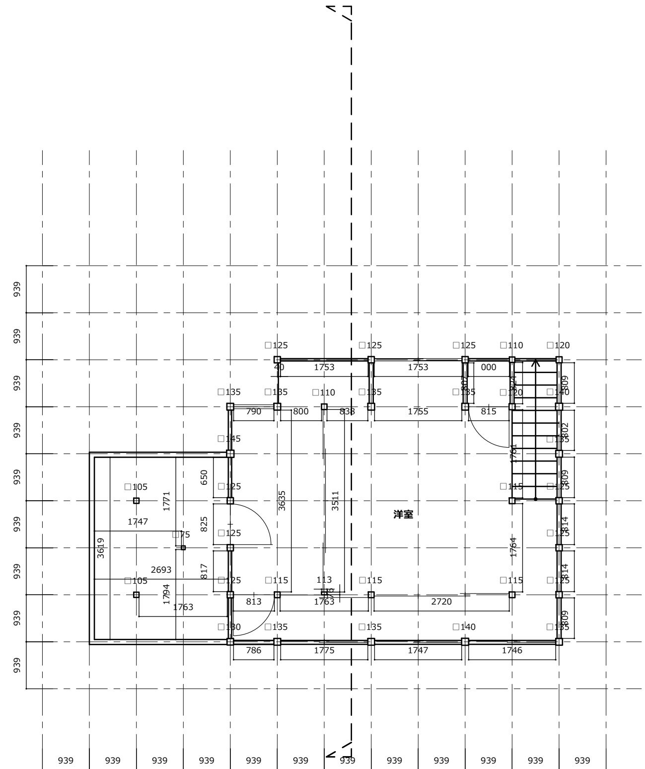
2階平面図
