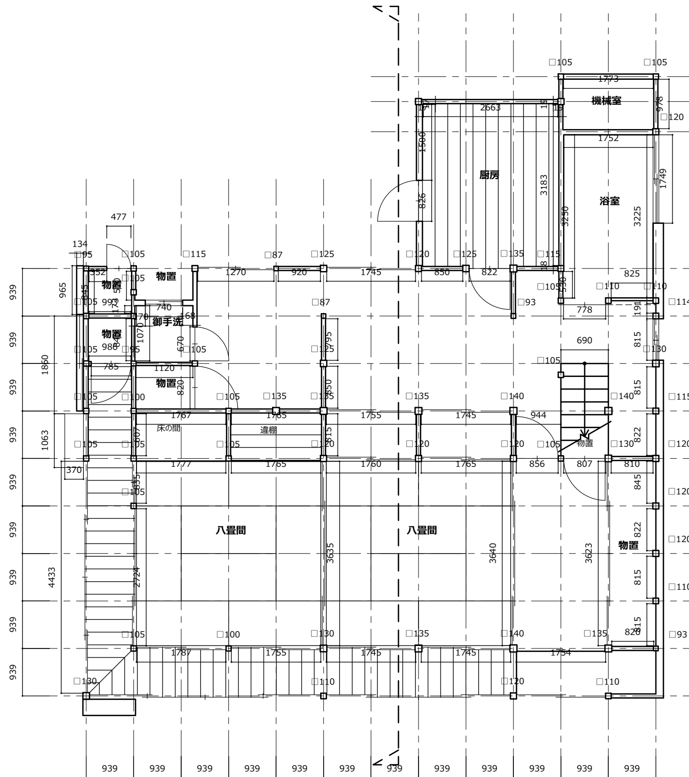
1階平面図
